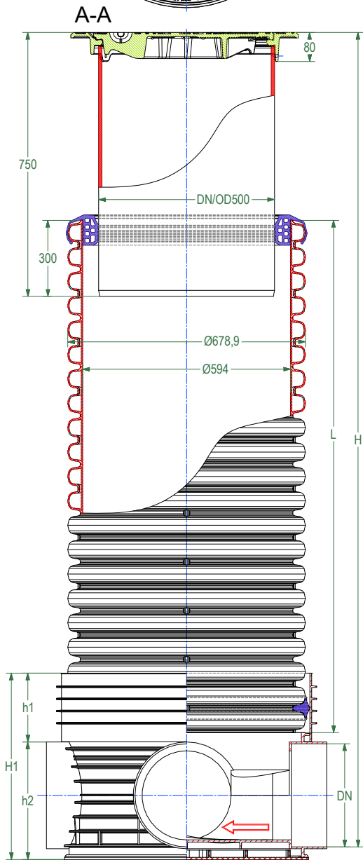
Akas pamatnes DN600, tips 3BL
