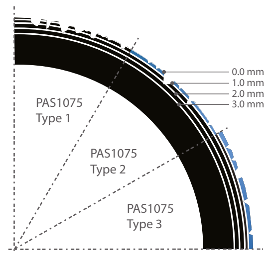
Caurules ārējās virsmas noturības salīdzinājums pret bojājumiem tādiem, kā skrāpējumi un skrambājumi ar un bez ārējās virsmas aizsardzības tādas, kā aizsargapvalka pārklājuma slānis.
