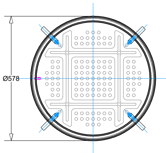
filtra trauks virsskats
